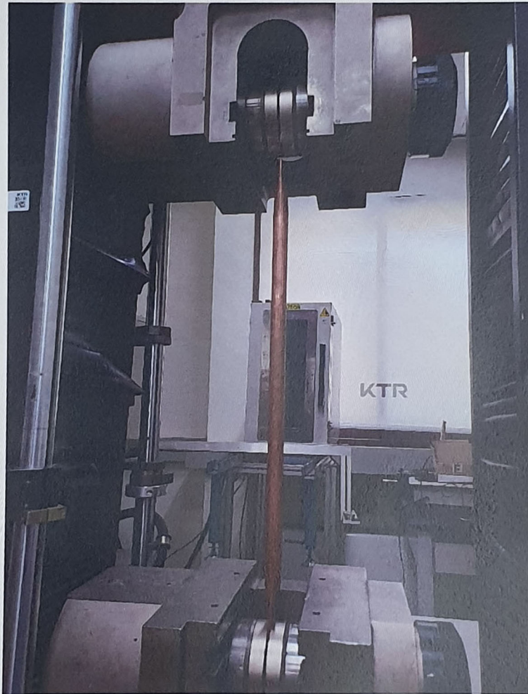
Tensile load test
